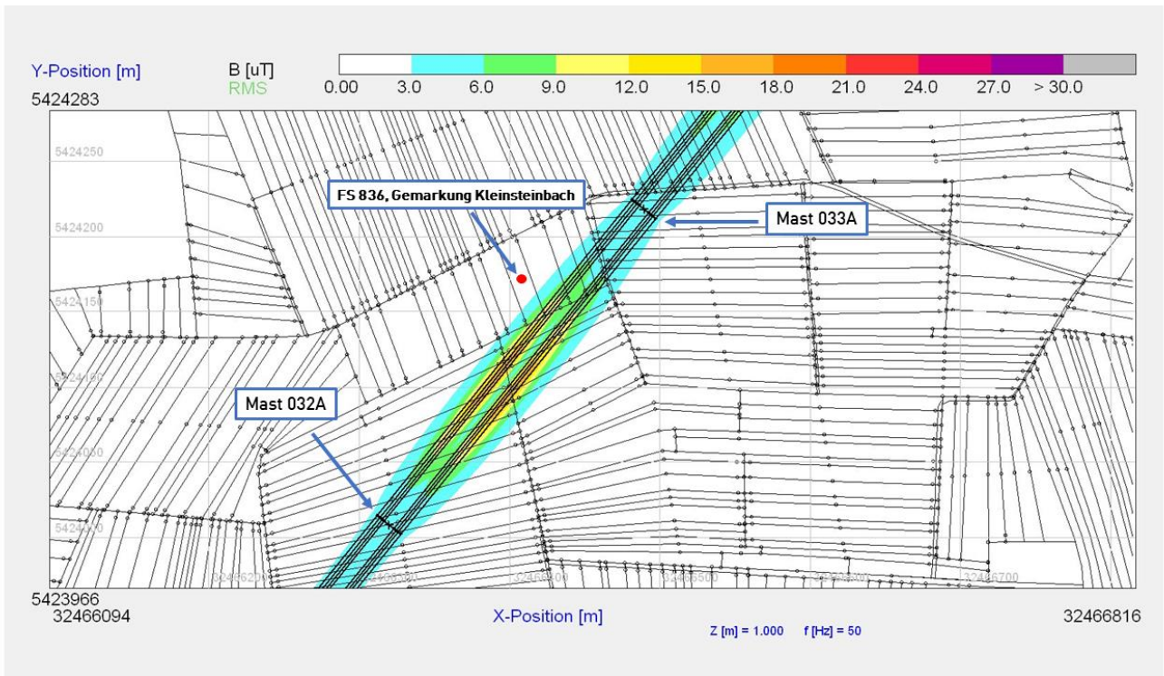
Abbildung 3: Magnetische Flussdichte im Spannfeld mit dem höchst exponierten Immissionsort (FS 836, Gemarkung Kleinsteinbach) zwischen Mast 032A und Mast 033A, Berechnungshöhe z=1 m
