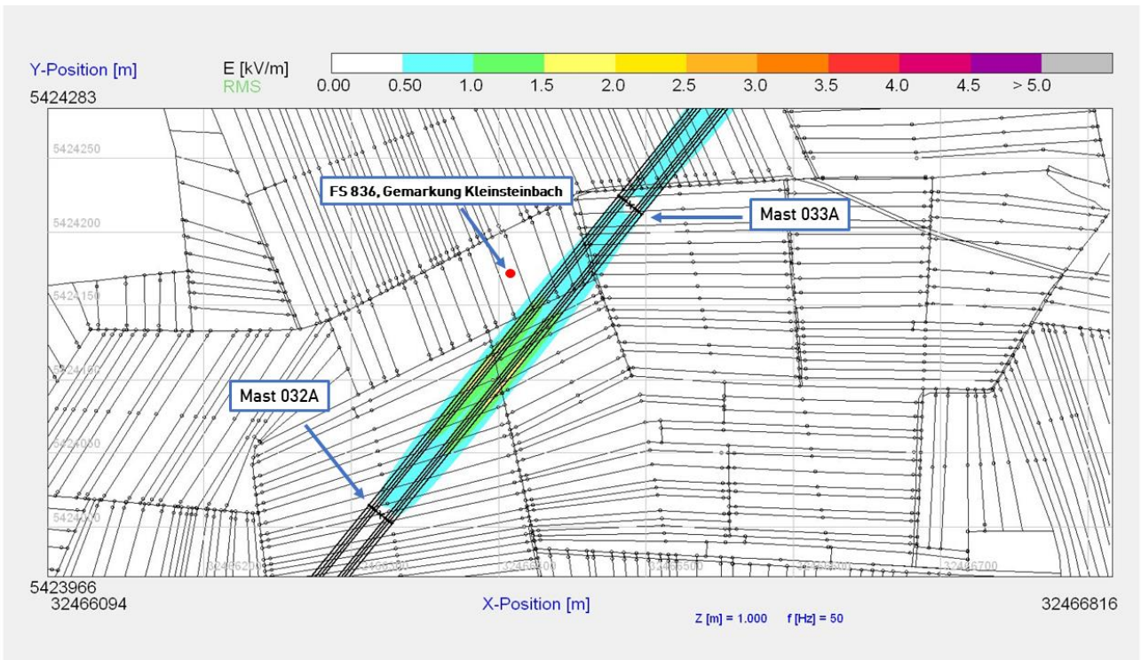
Abbildung 2: Elektrische Feldstärke im Spannfeld mit dem höchst exponierten Immissionsort (FS 836, Gemarkung Kleinsteinbach) zwischen Mast 032A und Mast 033A, Berechnungshöhe z=1 m
