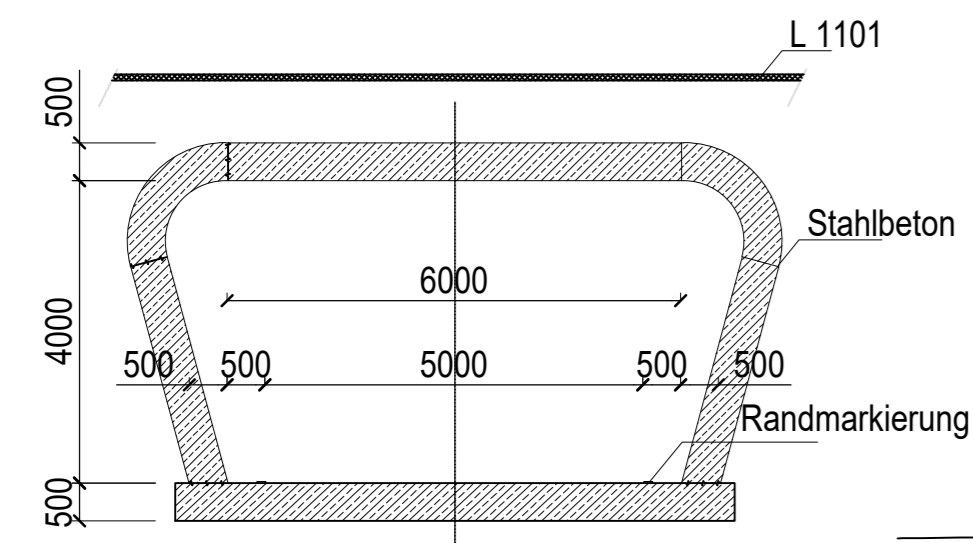
Querschnitt M1 : 100
