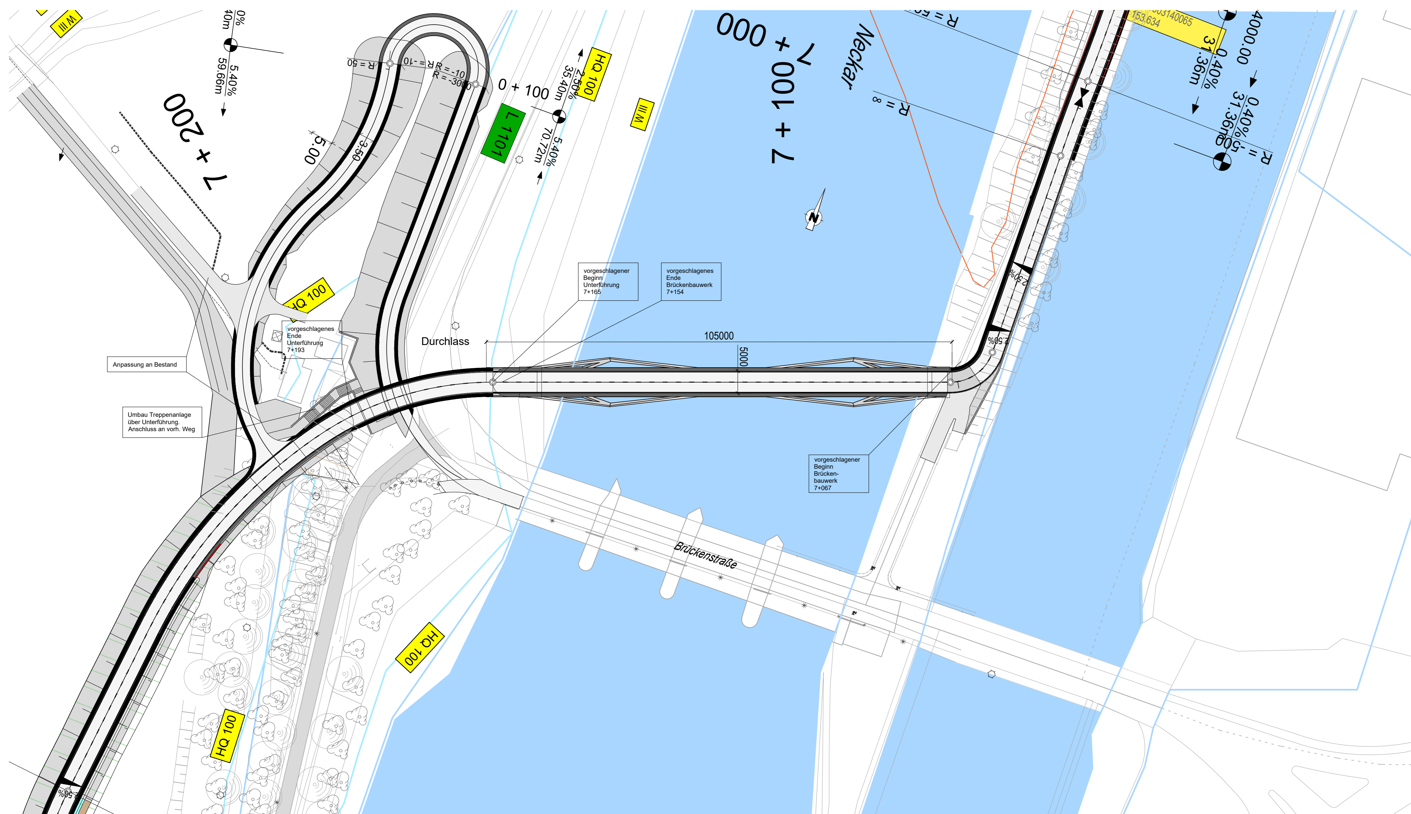
Lageplan M 1 : 500
