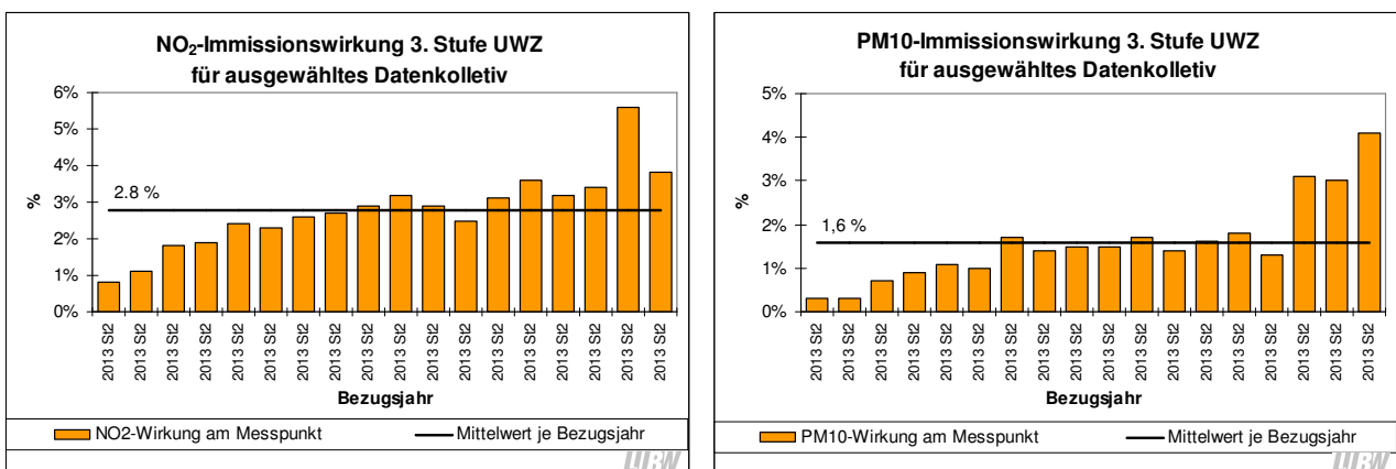
Abbildung 4-2: Relative Immissionswirkung der dritten Stufe der Fahrverbote an ausgewählten Messpunkten für \text{NO}_2 und \text{PM}_{10}
