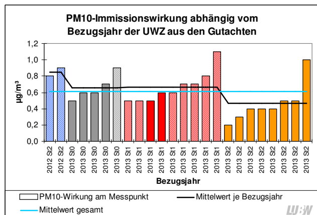
Abbildung 3-2: Immissionswirkung der Fahrverbote an ausgewählten Messpunkten für NO 2 und PM 10 in Abhängigkeit von den berechneten Bezugsjahren aus den Einzelgutachten, für die schraffierten Immissionswirkungen wird eine Anpassung des Bezugsjahres durchgeführt
