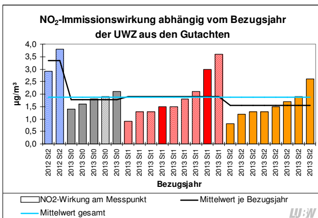
Abbildung 3-2: Immissionswirkung der Fahrverbote an ausgewählten Messpunkten für NO 2 und PM 10 in Abhängigkeit von den berechneten Bezugsjahren aus den Einzelgutachten, für die schraffierten Immissionswirkungen wird eine Anpassung des Bezugsjahres durchgeführt
