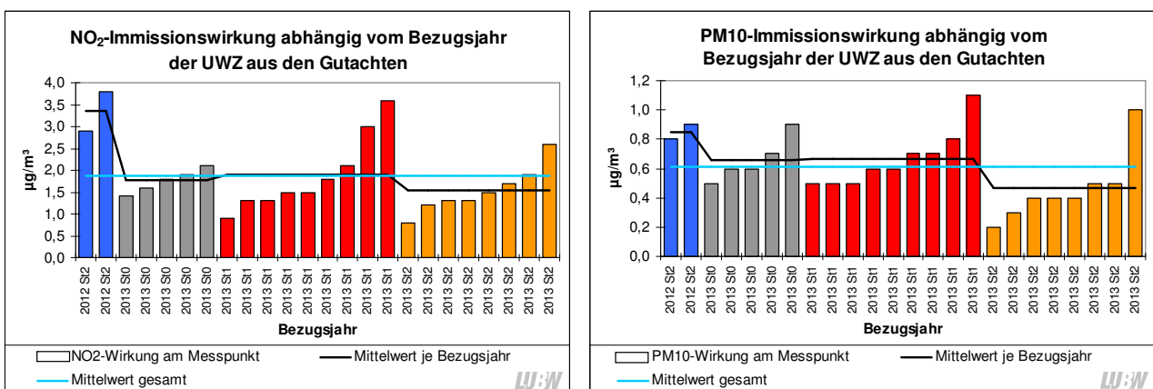
Abbildung 3-1: Immissionswirkung der Fahrverbote an ausgewählten Messpunkten für \text{NO}_2 und \text{PM}_{10} in Abhängigkeit von den berechneten Bezugsjahren aus den Einzelgutachten
