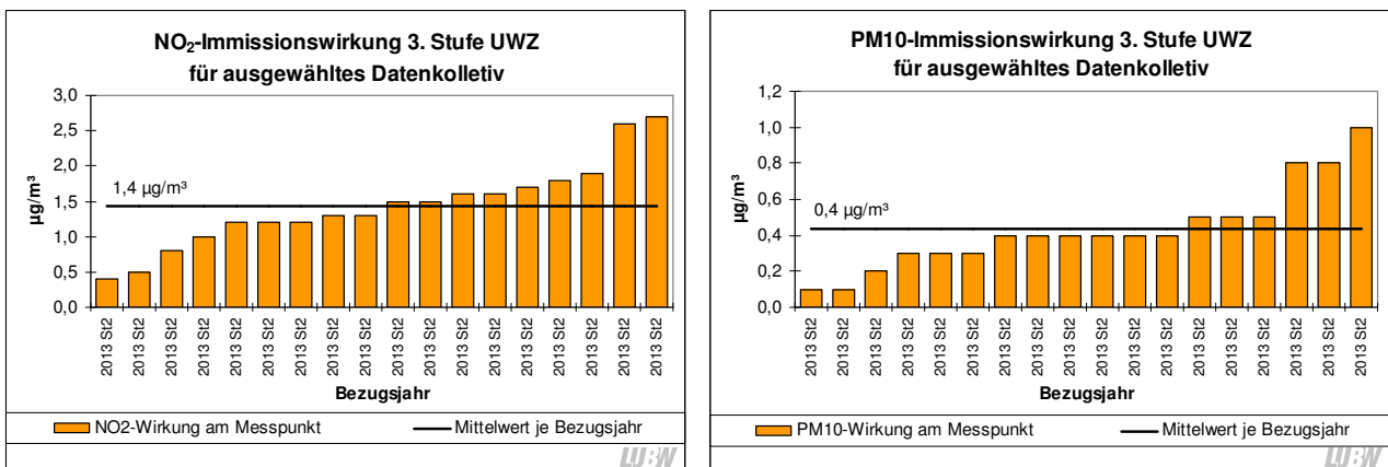
Abbildung 4-1: Immissionswirkung der dritten Stufe der Fahrverbote an ausgewählten Messpunkten für \text{NO}_2 und \text{PM}_{10}
