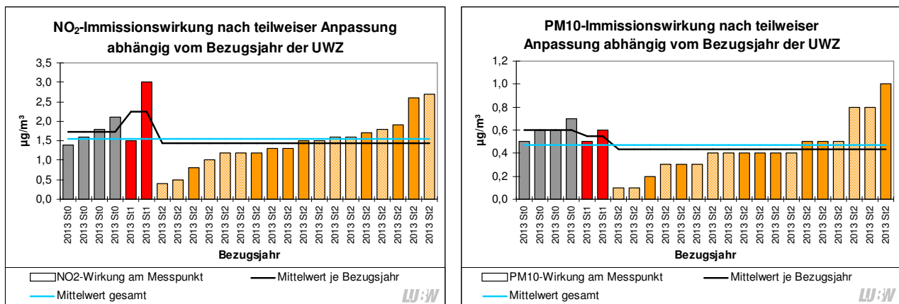
Abbildung 3-3: Immissionswirkung der Fahrverbote an ausgewählten Messpunkten für NO 2 und PM 10 nach Anpassung des Bezugsjahres, schraffierte Immissionswirkungen wurden angepasst
