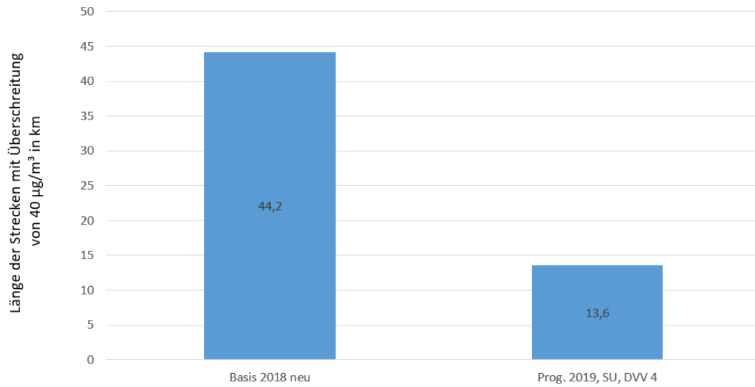
NO 2 -Immissionen 2018 und 2019, Stadtgebiet Stuttgart
