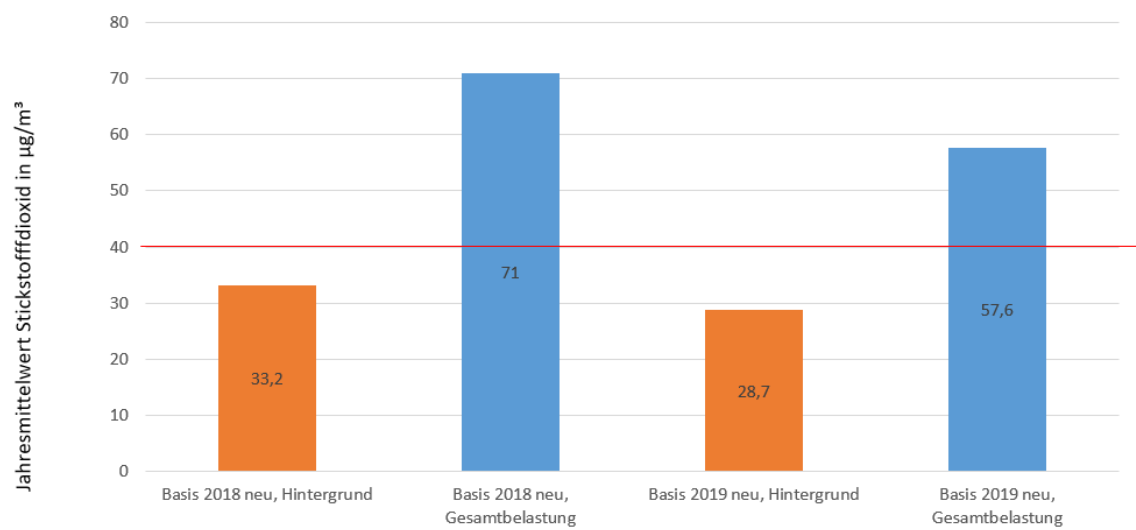
NO 2 -Immissionen 2018 und 2019, Station Am Neckartor
