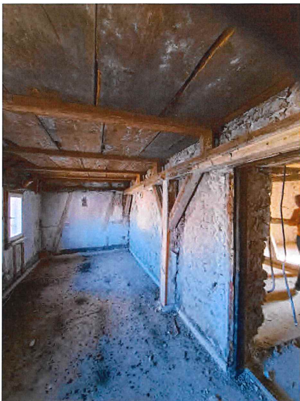
Fachwerkanbau - Innenhöhen max. 2,00 m
