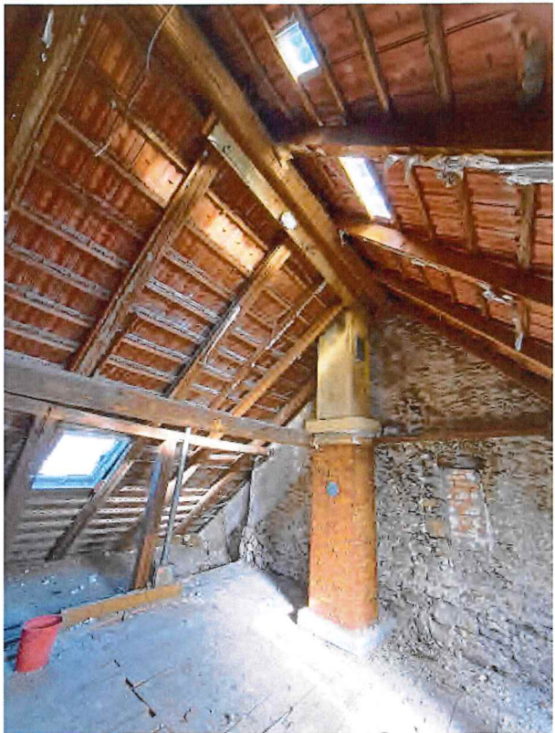
bestehender Dachstuhl → mehrfach umgebaut, Dachneigung Richtung Fachwerkanbau abgeändert
