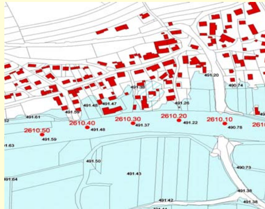
Überflutungen bei HQ 100 vor Bau
