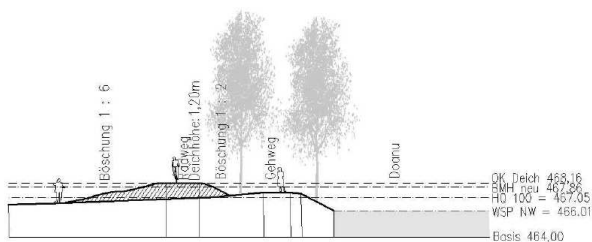
Musterquerschnitt Neuer Deich
