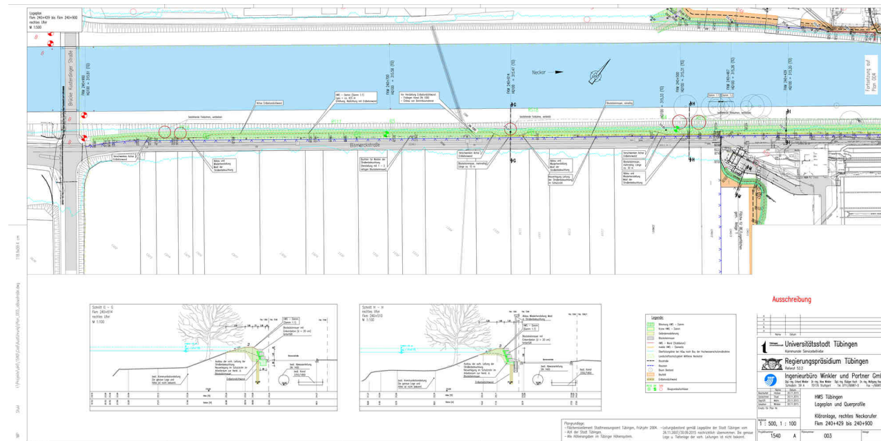
Abbildung Lageplan Dammertüchtigung rechtes Ufer
