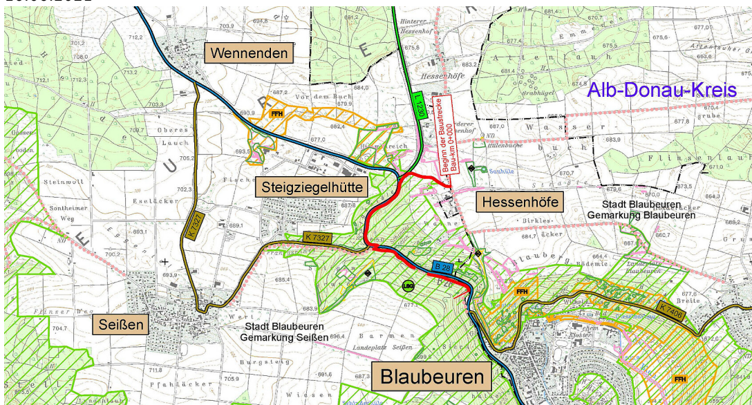
Übersichtslageplan zum Radweg Blaubeurer Steige Bauabschnitt II
