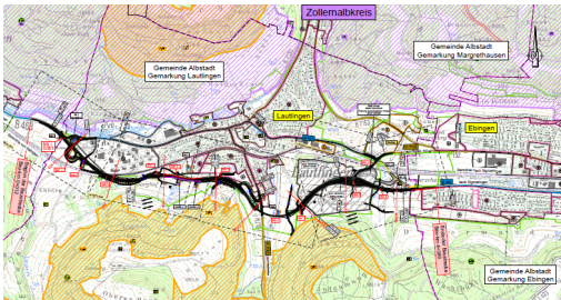
Übersichtsplan B463 Ortsumfahrung Lautlingen
