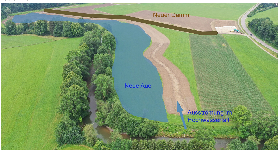
Geplante Hochwasserschutzmaßnahme in Hiltensweiler
