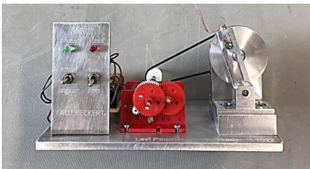
Elektrisch angetriebene Kurbelschwinge
