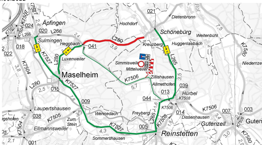
Lageplan Umleitungsskizze L 280 Heggbach - Schönebürg
