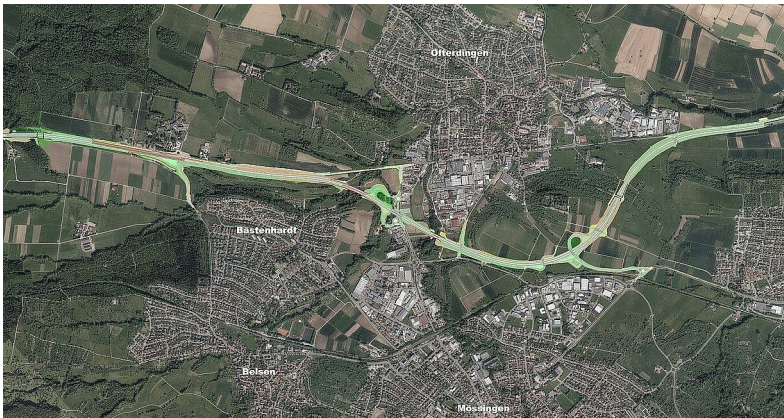
Lageplan des geplanten zweibahnigen Ausbau der B 27 zwischen Bodelshausen und Nehren
