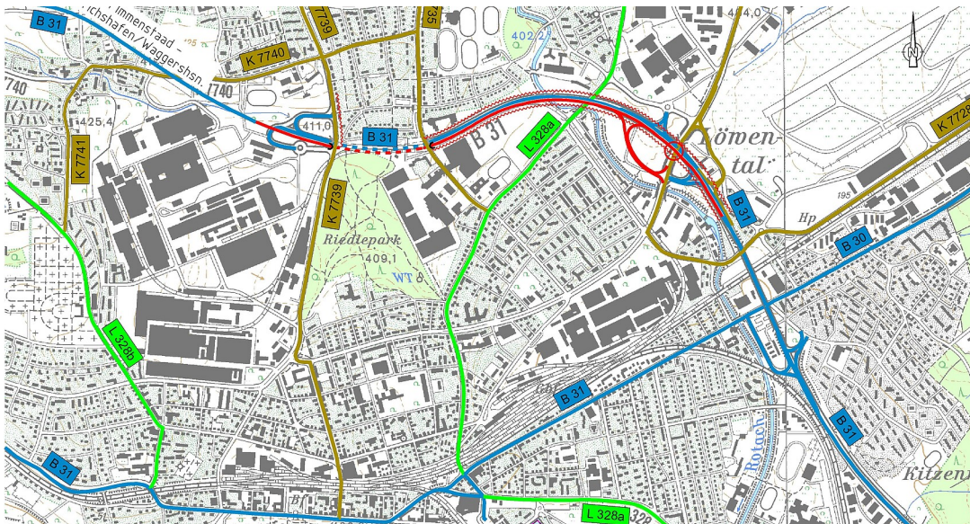
Übersichtslageplan Ausbau der B 31 zwischen dem Tunnel Waggershausen und dem Löwentalknoten in Friedrichshafen
