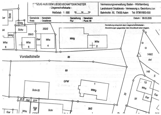
Lageplan, 73450 Neresheim (Härtsfeld), Vorstadtstraße 1
