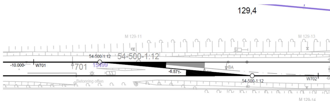
Abbildung 16: Gleisverbindung W701/W702
