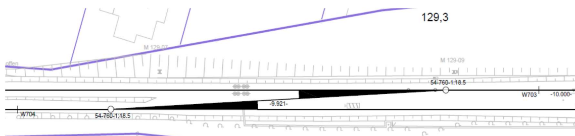
Abbildung 17: Gleisverbindung W703/W704
